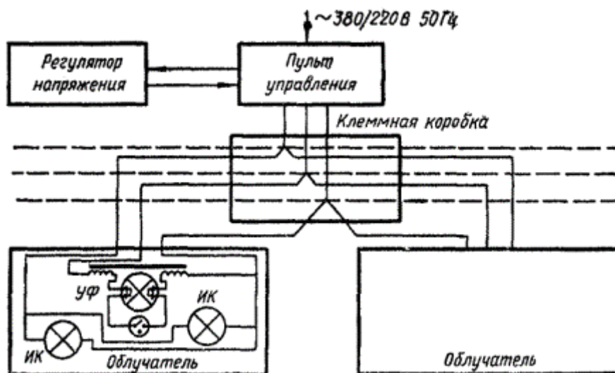
Рис. 8. Структурная электрическая схема установки «Луч».
