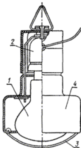
Рис. 4. Инфракрасный облучатель ОВИ-1:
