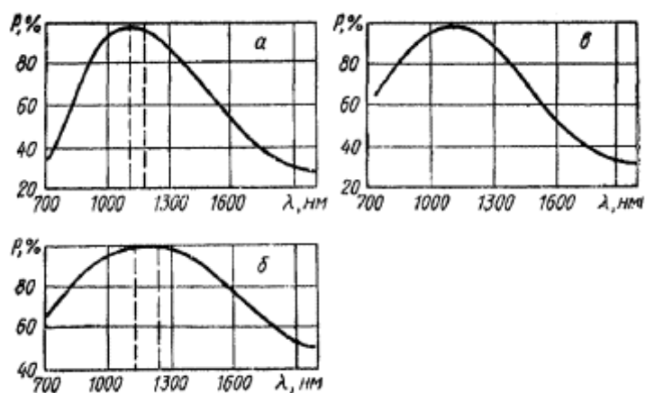
Рис. 1. Относительное распределение спектральной интенсивности излучения инфракрасных ламп:
