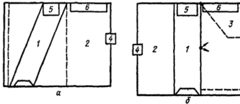
Рис. 13. Схемы устройства станков для проведения опоросов и выращивания поросят под матками:
