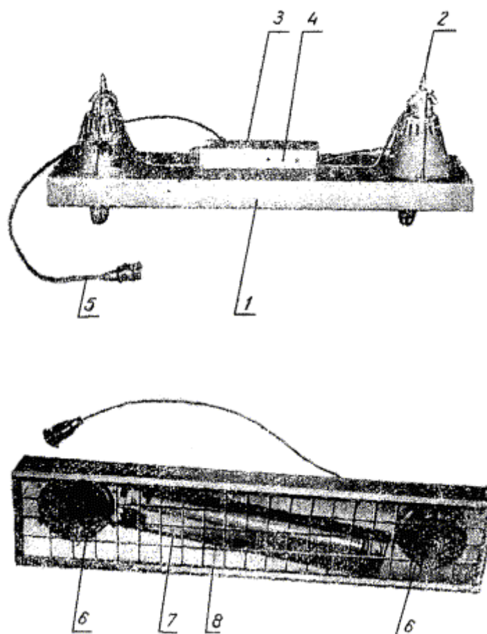
Рис. 6. Облучатель установки ИКУФ-1:
